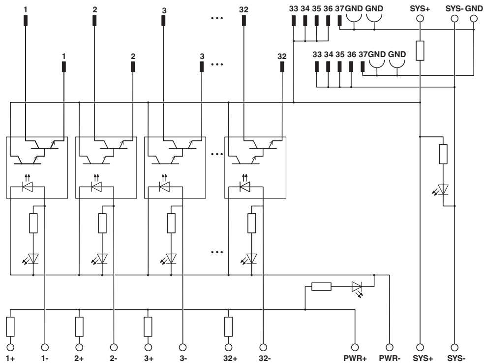
Diagrama eléctrico
