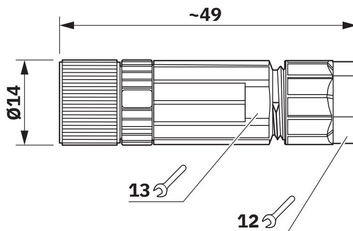
Dessin coté
