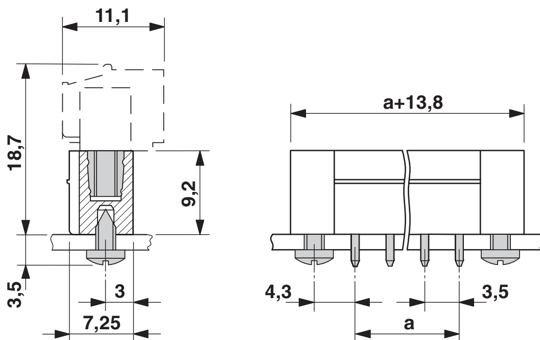
Dessin coté
