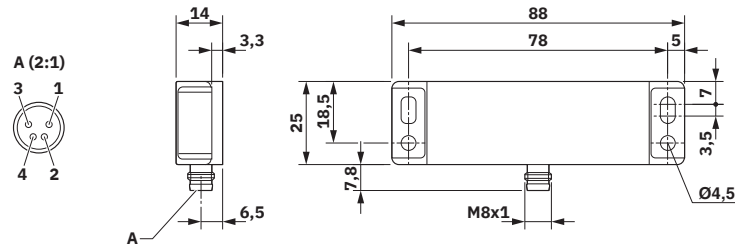
Dessin coté
