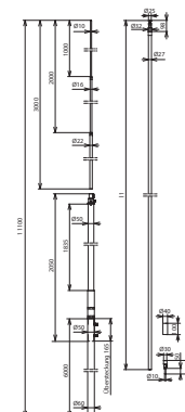
Maßbild FM 60 L11M IP HVIP L10M GFK AL
