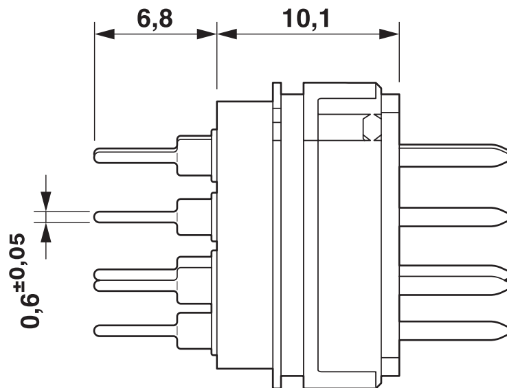
Dessin coté
