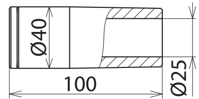
Maßbild SRA NS
