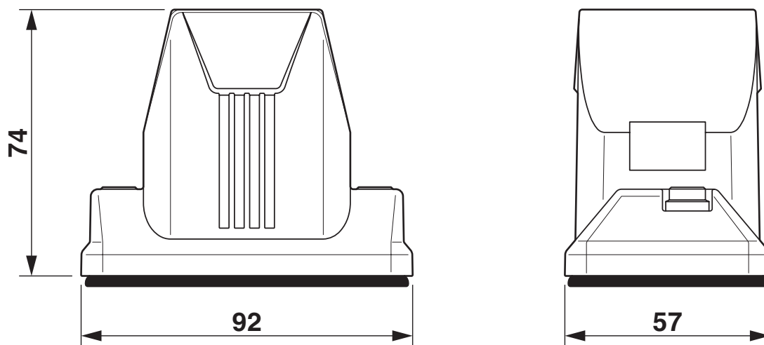
Maßzeichnung
