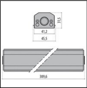
3107575 Kit box di alimentazione DALI IN / OUT L500
