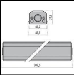
3107574 Kit box di alimentazione DALI IN L500
