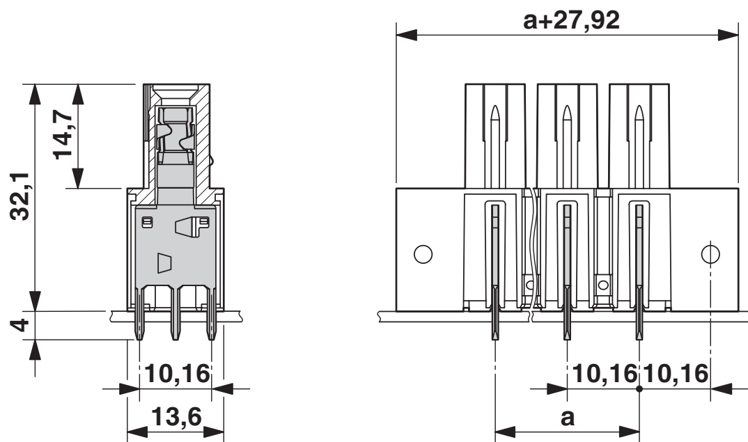
Dessin coté
