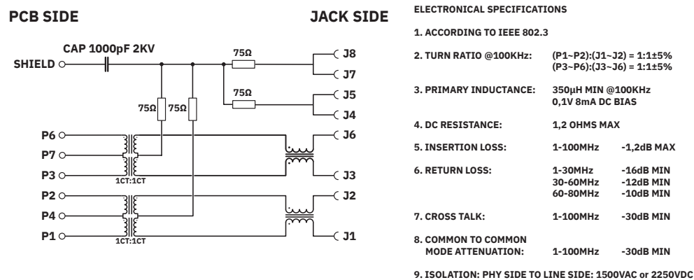
Diagrama eléctrico
