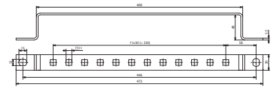
Maßbild ES 12AP 11X11 V2A
