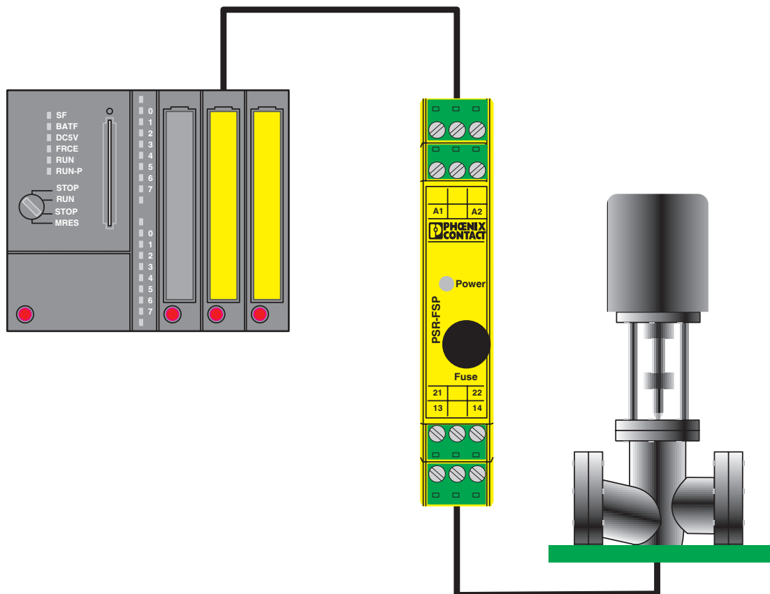
Applikationszeichnung
