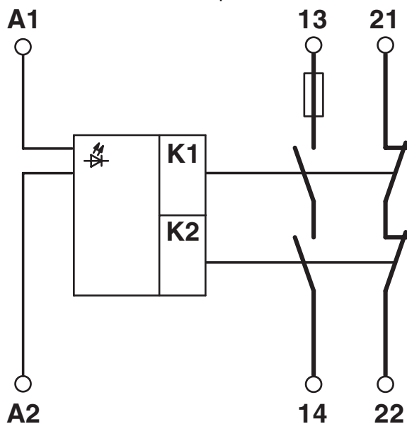
Schaltplan
