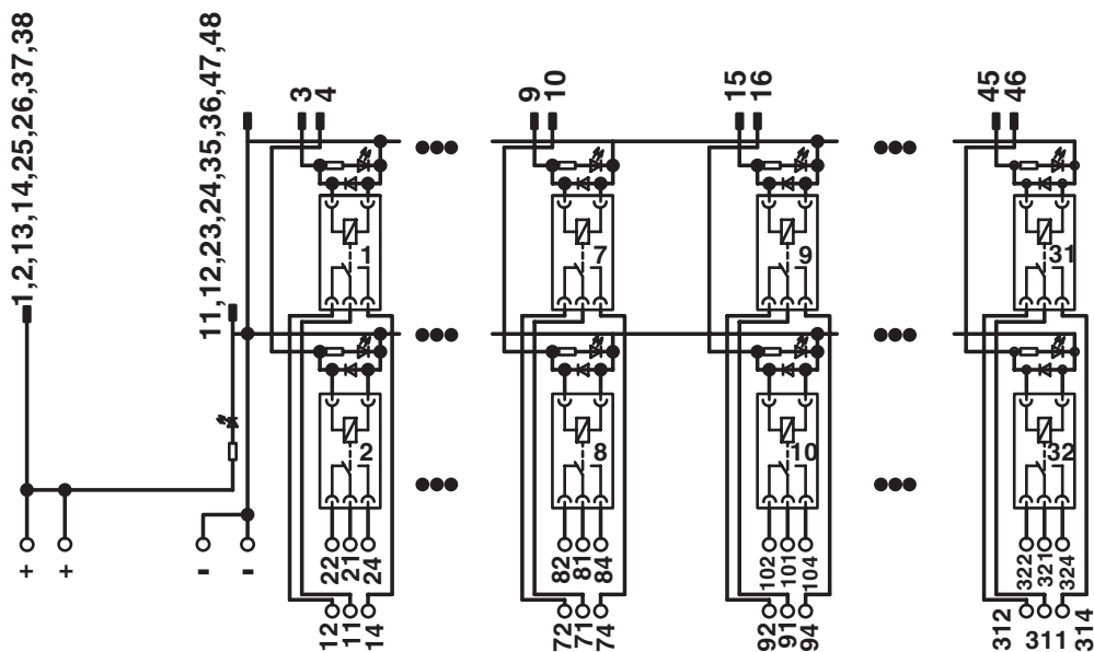
Diagrama eléctrico
