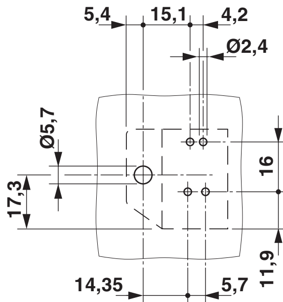
Bohrplan/Lötpadgeometrie
