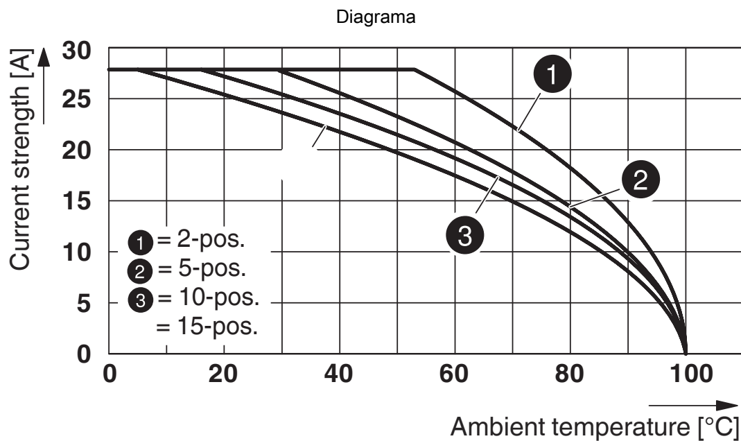
Diagrama eléctrico
