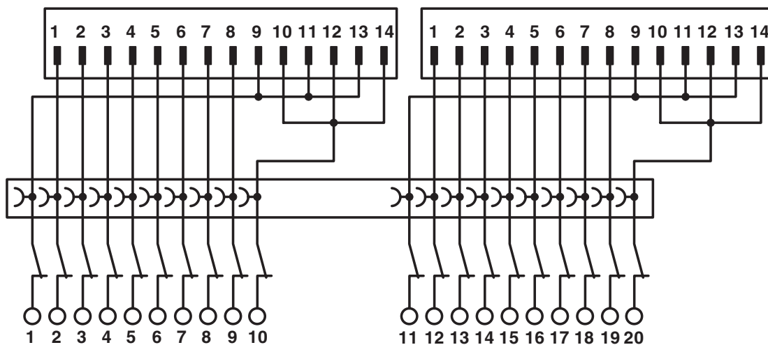
Esquema de conexiones FLKM-2FLK14/KDS3-MT/PPA/S7
