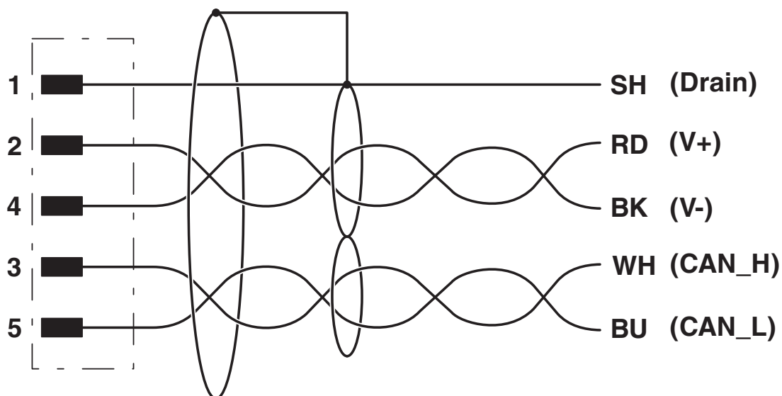
Diagrama eléctrico
