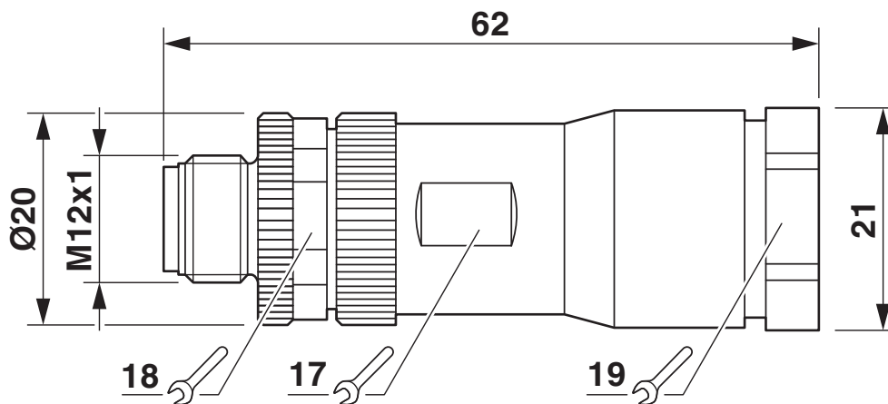
Maßzeichnung
