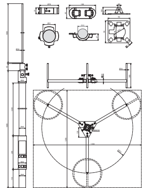
Maßbild FM D40 L2700 GFK AL V2A DBS
