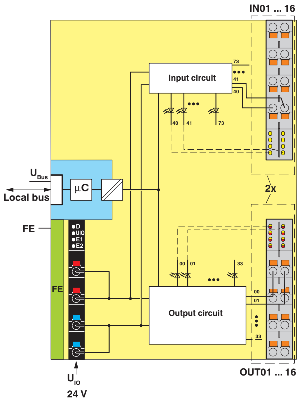
Schéma fonctionnel
