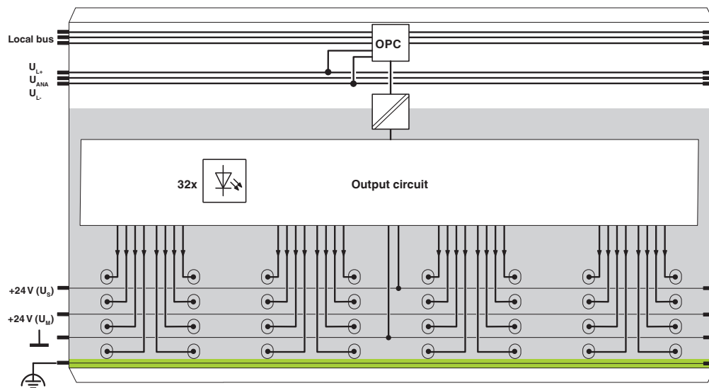
Schéma fonctionnel
