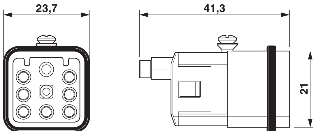
Stifteinsatz (gedrehte Kontakte)
