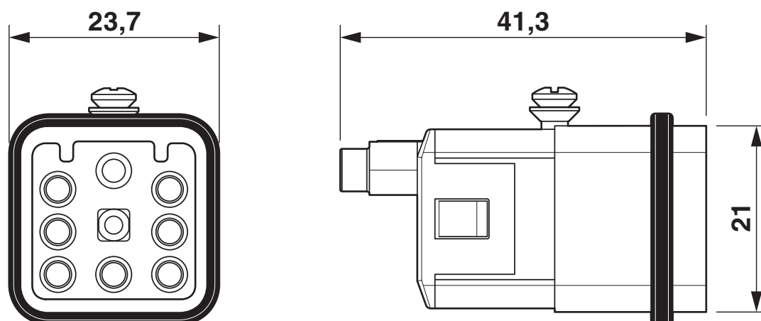
Inserto de machos (contactos mecanizados)
