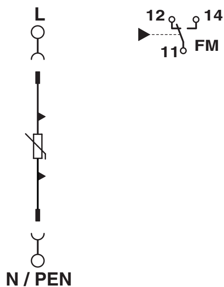
Schaltplan
