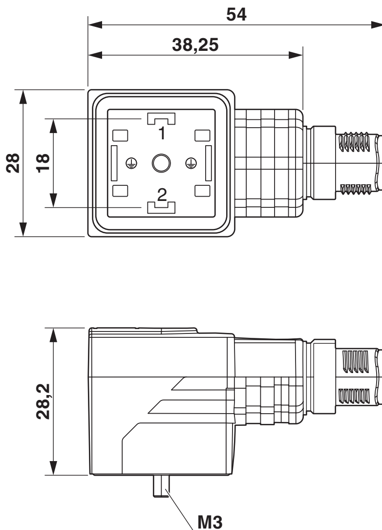
Dessin coté
