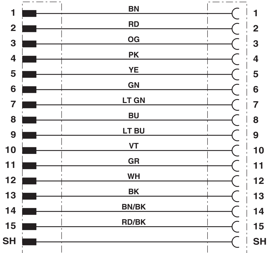
Schaltplan
