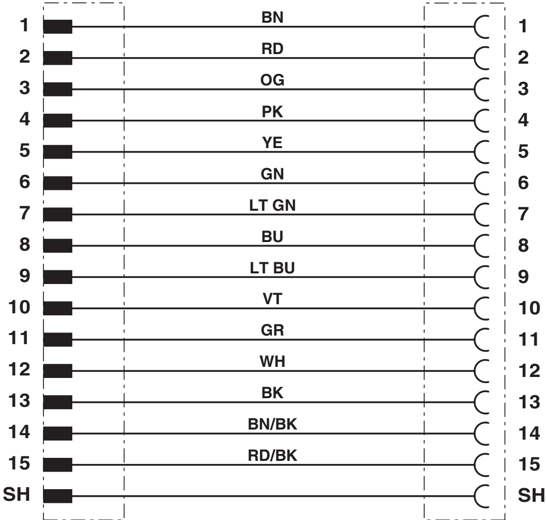
Diagrama eléctrico
