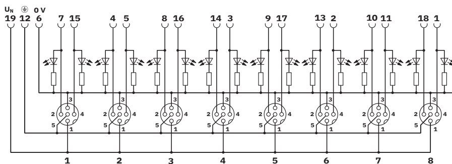
Diagrama eléctrico
