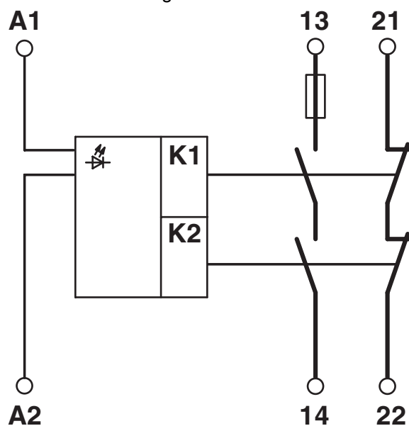
Diagrama eléctrico
