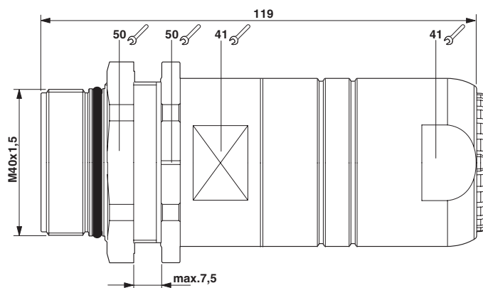
Maßzeichnung
