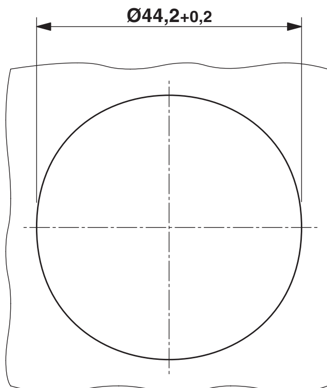
Dessin coté
