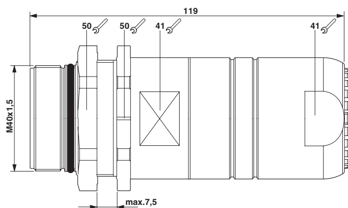
Dessin coté
