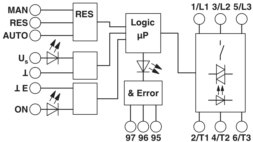
Schéma fonctionnel
