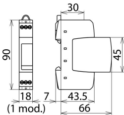
Dimensiones del DR M 2P 60
