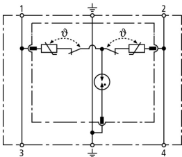
Esquema del DR M 2P 60
