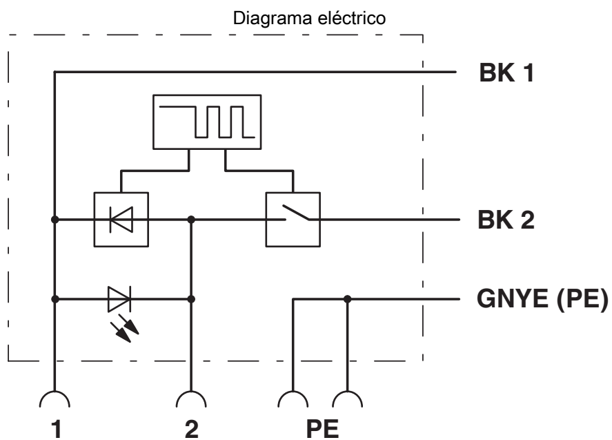
Ocupación de contactos del conector de válvula
