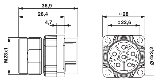
Dessin coté
