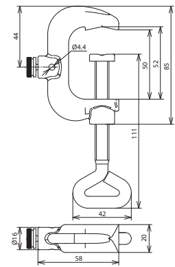
Maßbild PK 4.45 ASSM5 TGTZN
