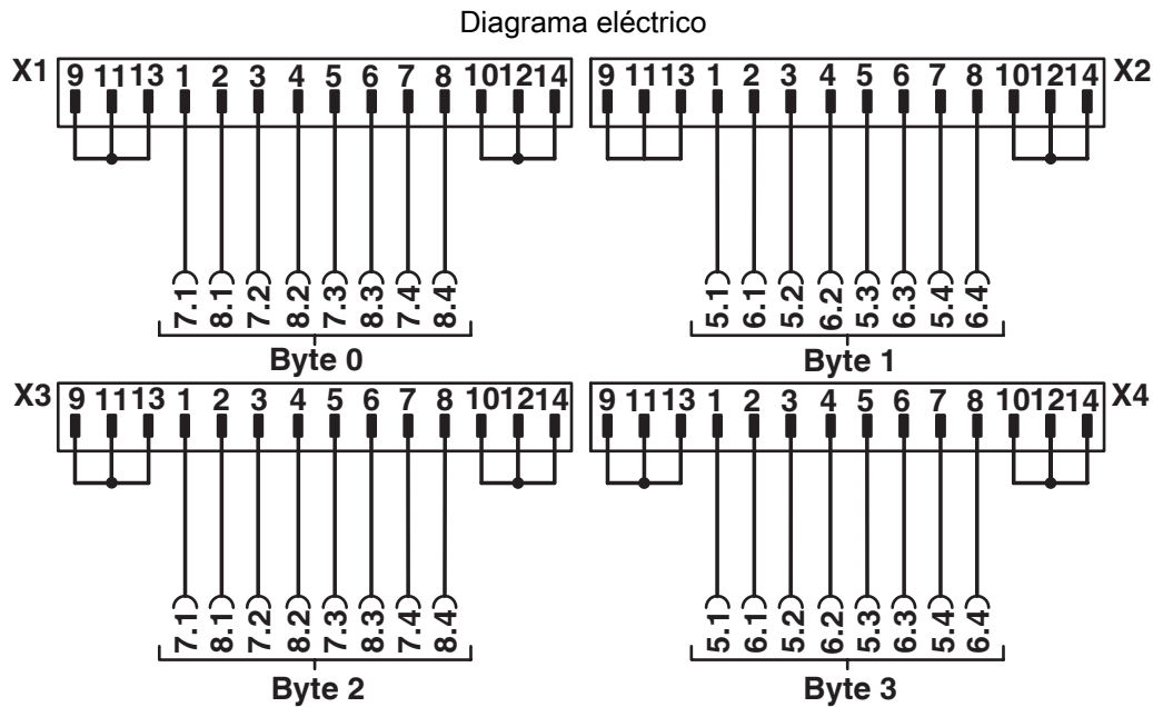
Esquema de conexiones FLKM 14-PA-INLINE/32
