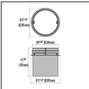
3111135 Einbautopf
