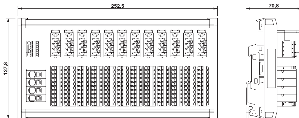
Dessin coté
