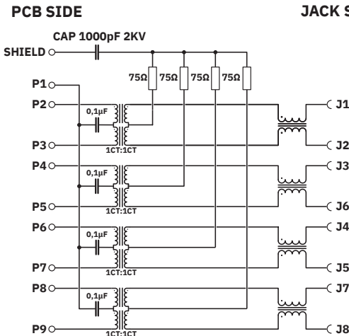
Schaltplan
