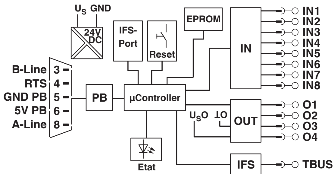
Schéma fonctionnel
