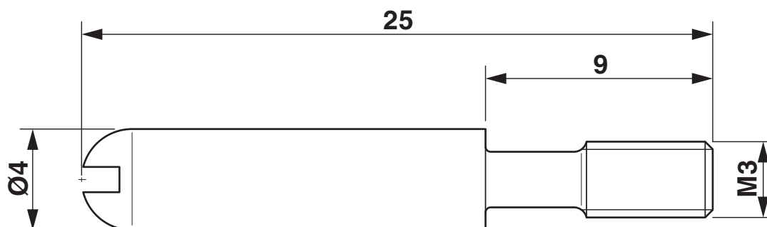
Dessin coté
