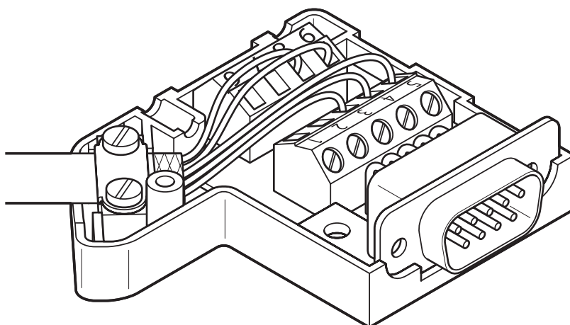
Dessin schématique
