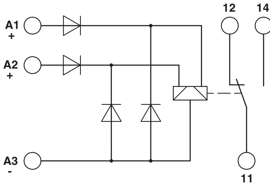
Schaltplan
