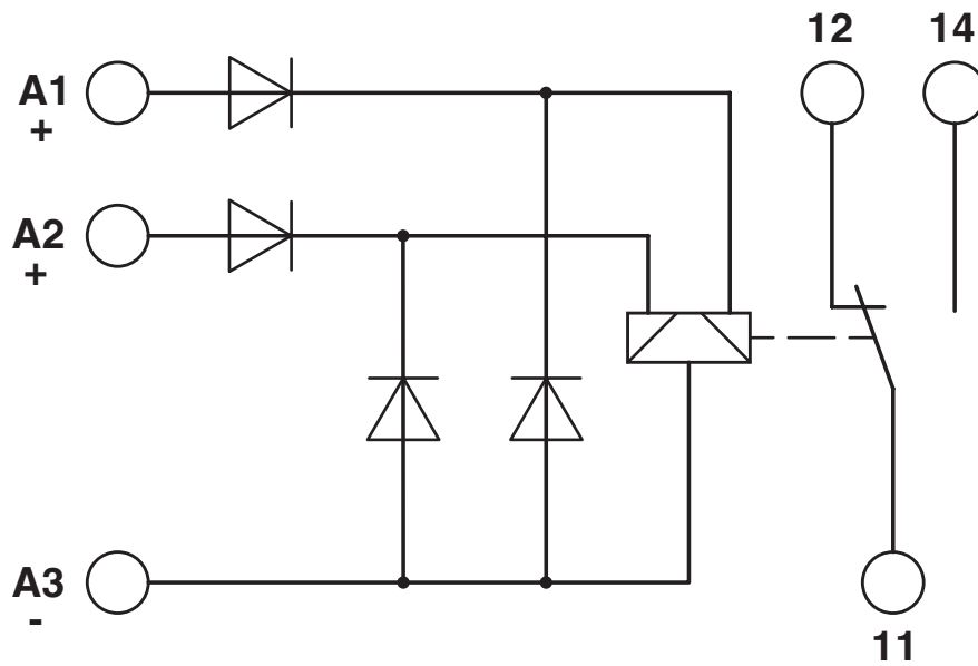
Diagrama eléctrico
