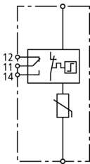
Esquema del DG 1000 FM
