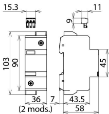
Dimensiones del DG 1000 FM
