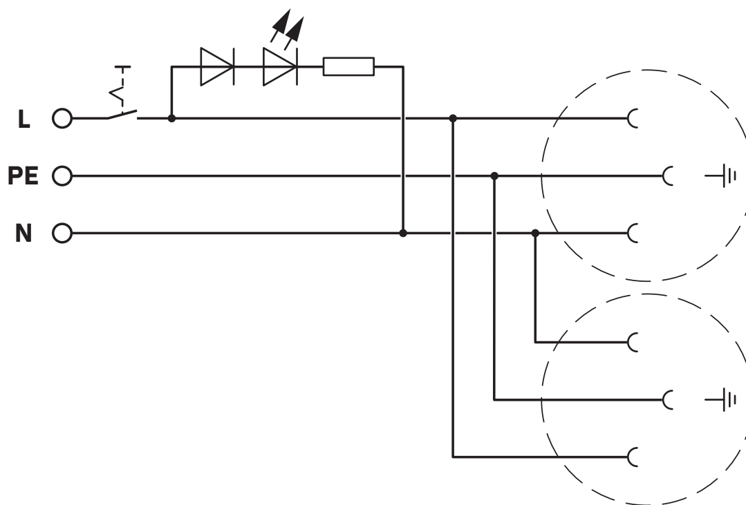
Schaltplan
