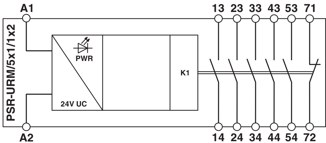
Schéma fonctionnel
