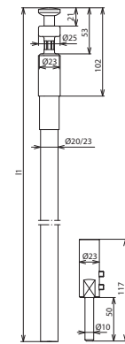
Maßbild HVI RIV 75 23 L6M GR M
